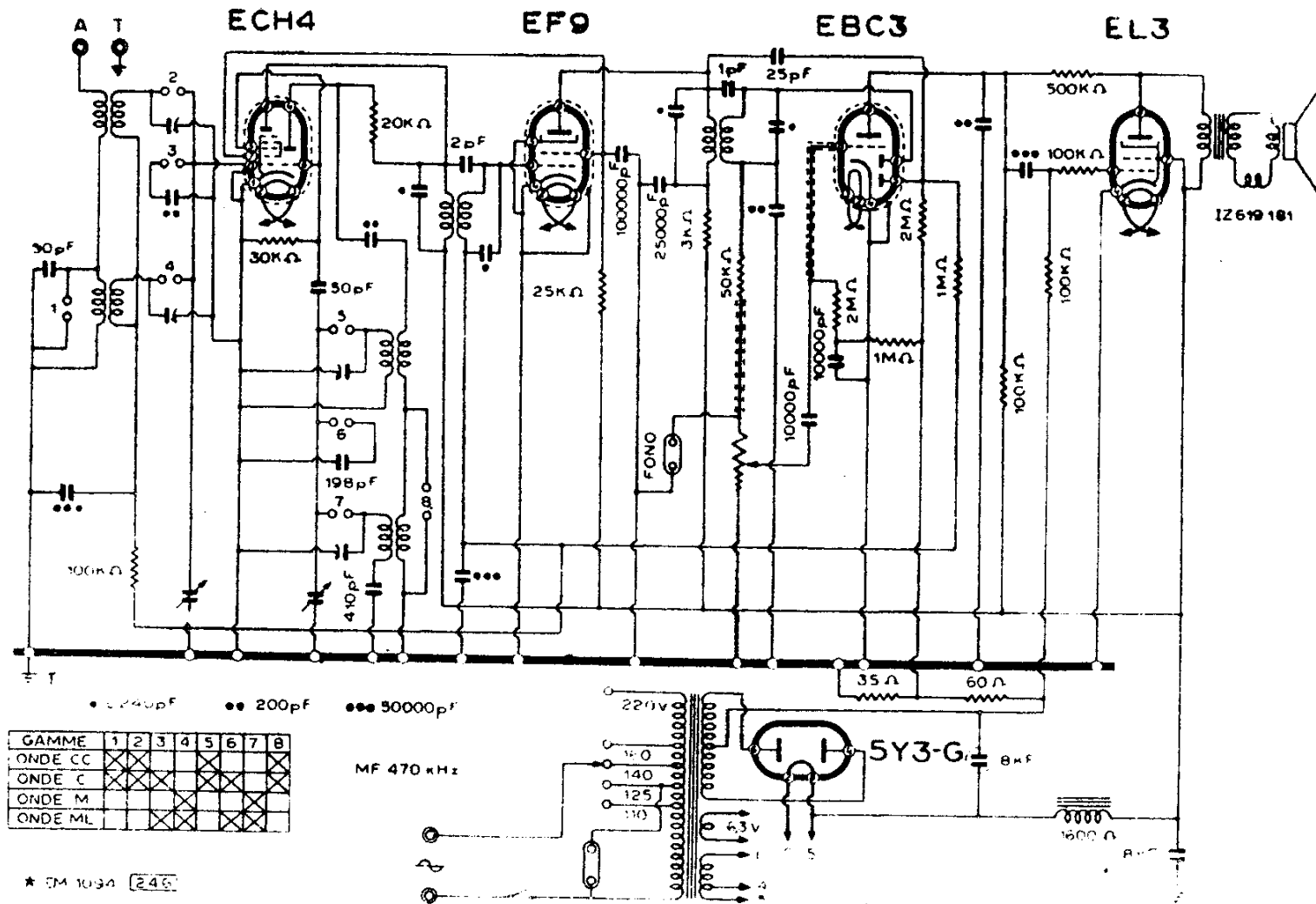
F.I.M.I. - MOD. PHONOLA « 585 »
